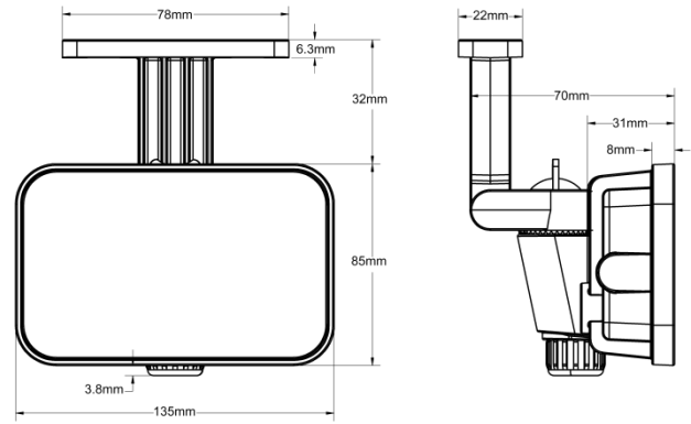
Desenho Técnico - 30W
