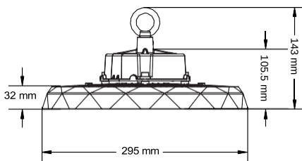
Τεχνικό Σχέδιο
