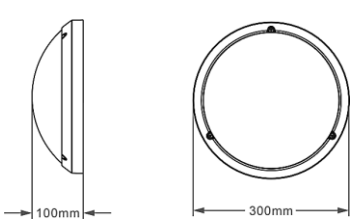
Τεχνικό Σχέδιο
