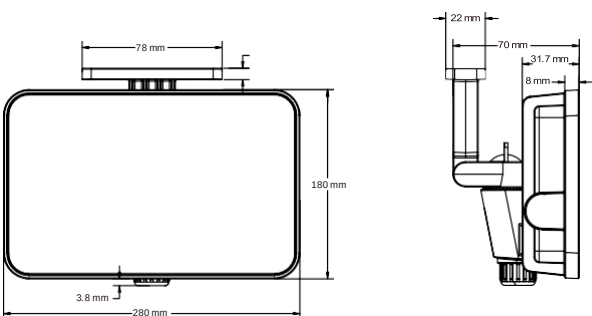
Τεχνικό σχέδιο - 100W
