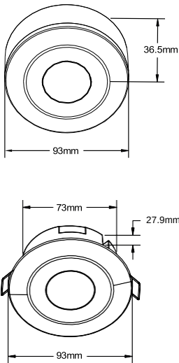
Τεχνικό Σχέδιο
