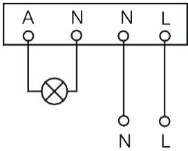
Διάγραμμα Σύνδεσης
