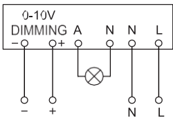
Διάγραμμα Σύνδεσης
