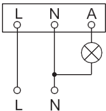
Διάγραμμα Σύνδεσης
