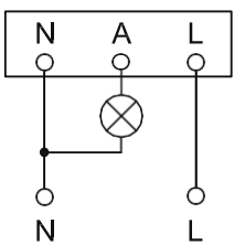
Διάγραμμα Σύνδεσης
