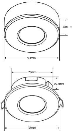
Τεχνικό Σχέδιο
