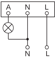
Διάγραμμα Σύνδεσης
