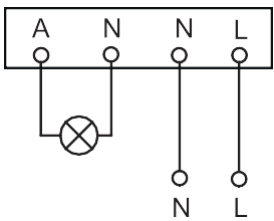
Διάγραμμα Σύνδεσης
