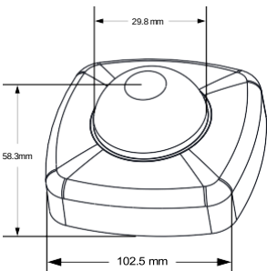
Τεχνικό Σχέδιο
