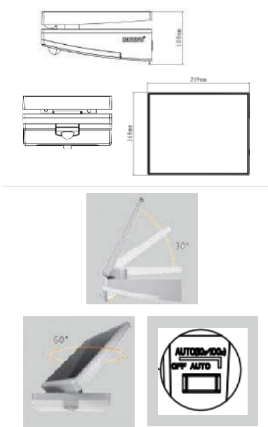
Τεχνικό Σχέδιο
