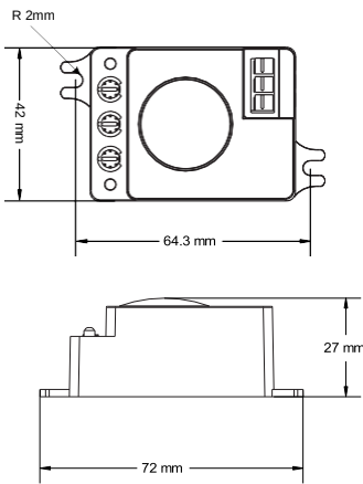
Τεχνικό Σχέδιο
