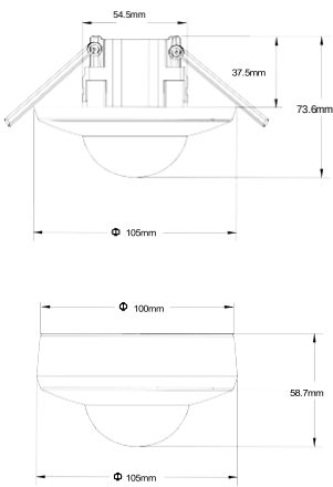
Τεχνικό Σχέδιο
