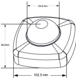
Τεχνικό Σχέδιο
