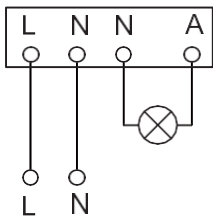
Διάγραμμα Σύνδεσης
