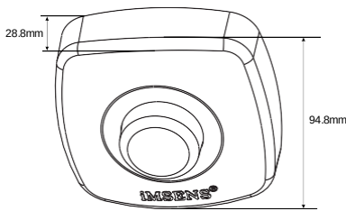
Τεχνικό Σχέδιο
