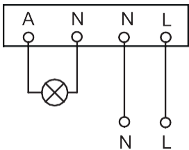
Διάγραμμα Σύνδεσης
