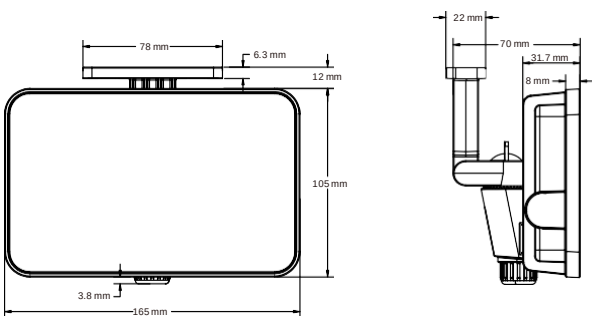
Τεχνικό σχέδιο - 50W
