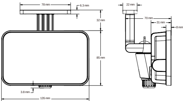
Τεχνικό σχέδιο - 20W
