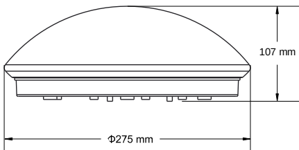
Τεχνικό Σχέδιο
