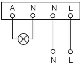
Διάγραμμα Σύνδεσης
