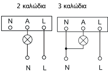
Διάγραμμα Σύνδεσης
