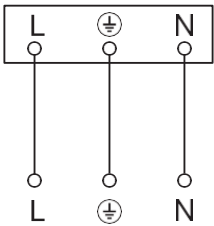
Διάγραμμα Σύνδεσης
