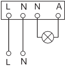
Διάγραμμα Σύνδεσης
