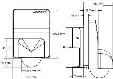
Τεχνικό Σχέδιο
