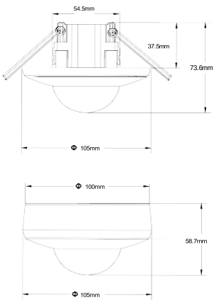
Τεχνικό Σχέδιο
