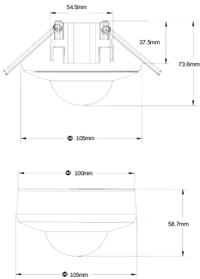
Τεχνικό Σχέδιο
