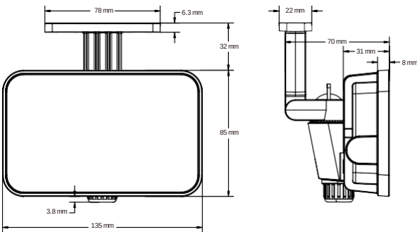
Τεχνικό σχέδιο - 30W
