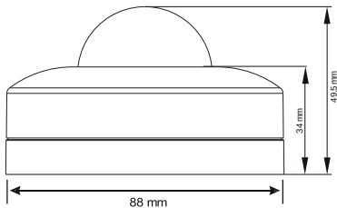
Τεχνικό Σχέδιο
