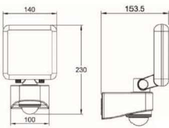
Τεχνικό Σχέδιο
