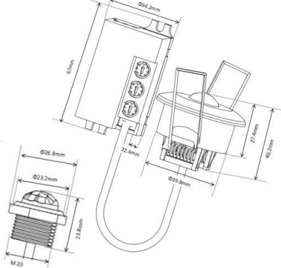
Τεχνικό Σχέδιο
