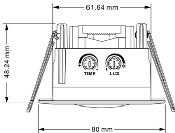
Τεχνικό Σχέδιο
