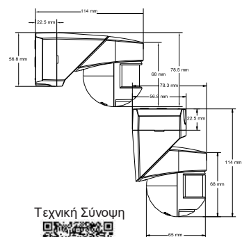
Τεχνικό Σχέδιο
