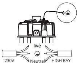
Διάγραμμα Σύνδεσης
