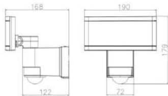
Τεχνικό Σχέδιο
