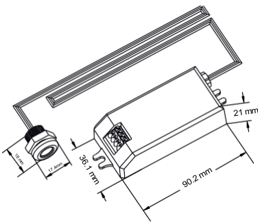
Τεχνικό Σχέδιο
