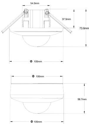
Τεχνικό Σχέδιο
