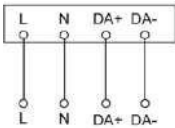
Διάγραμμα Σύνδεσης
