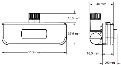
Τεχνικό Σχέδιο
