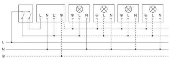
Diagrama de instalação através de um interruptor em série para o modo manual e automático
